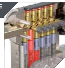
TRIPLE SYSTÈME ANTI-BUMPING
